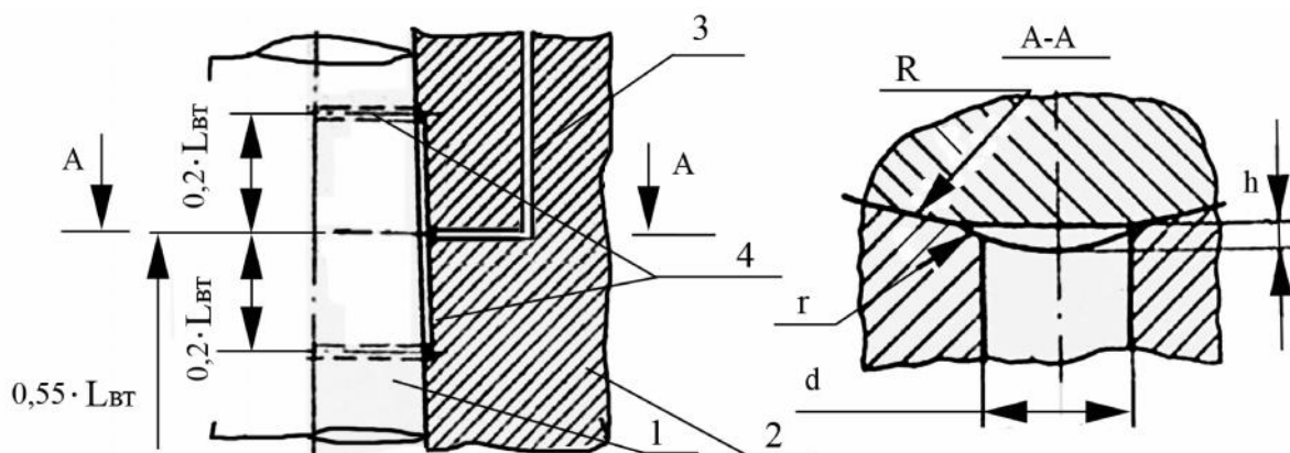
Рис. 15. Схема каналов подвода масла: 1 – баллер; 2 – румпель; 3 – маслоподводящие канавки; 4 – маслораспределительные канавки; L_{вт} – высота соединения; h – глубина канавки; R, r – радиус профиля канавок
