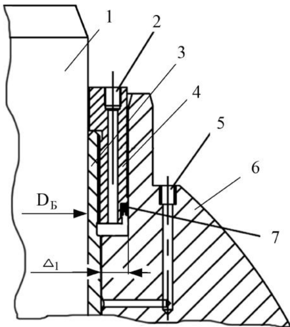
Рис. 17. К расчету давления насоса, обеспечивающего осевое перемещение ротора относительно баллера:
