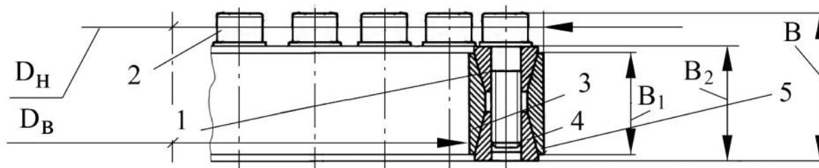
Рис. 11. Клиновое кольцо в сборе: 1, 4 – коническая втулка; 2 – винт; 3, 5 – разрезные конические кольца
