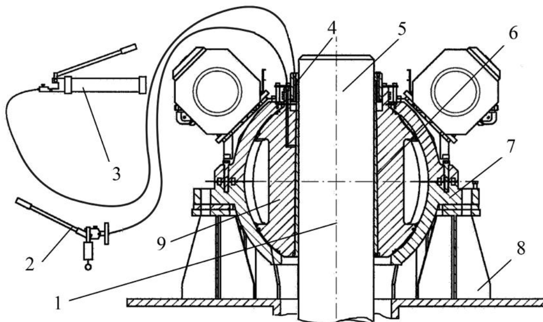
Рис. 13. Схема гидропрессового способа монтажа рулевой машины на баллере:
