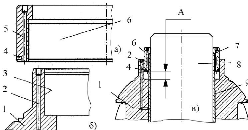
Рис. 14. Элементы гидропрессового соединения СРМ: 1 – ротор; 2 – канал подачи масла в зазор в соединении при запрессовке; 3 – поверхность контакта с подвижной гидрогайкой; 4 – прокладка; 5 – канал подачи масла для насаживания румпеля на баллер; 6 – гидравлическая гайка; 7 – упор гидрогайки; 8 – баллер; 9 – клиновидная втулка
