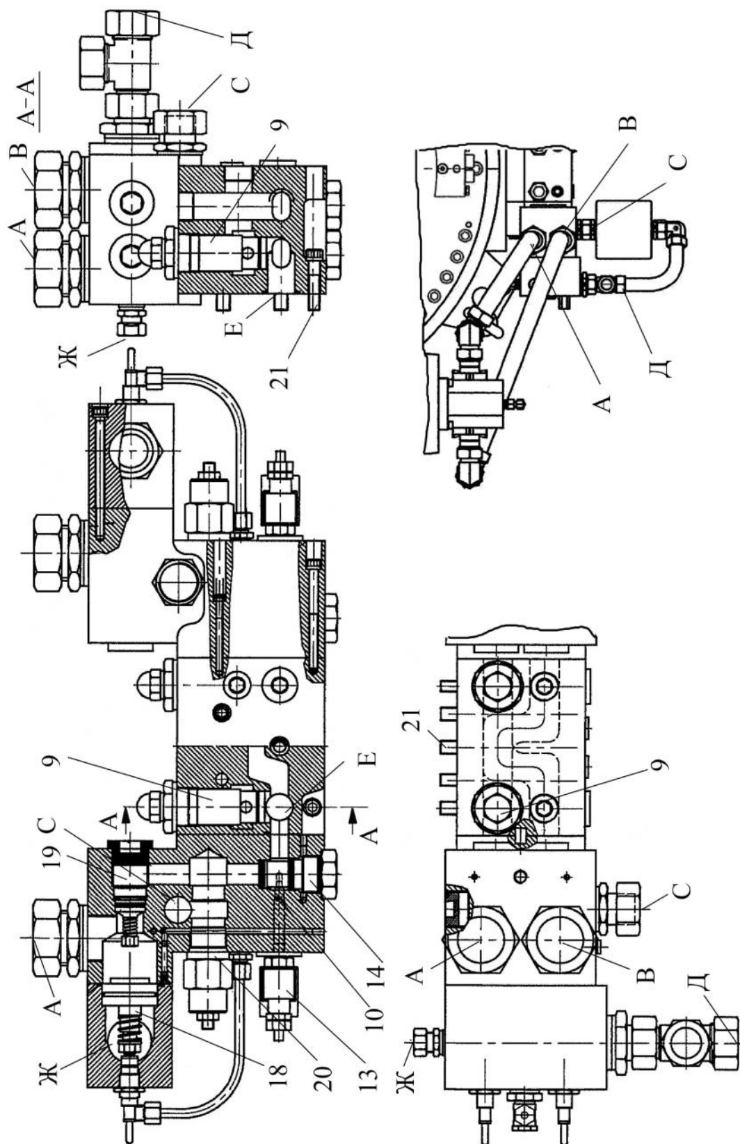
Рис. 9. Гидроблок: 9, 20 – предохранительный клапан (20 МПа); 10, 18, 19 – обратный клапан; 13 – гидрораспределитель; 14 – гидрораспределительный клапан
