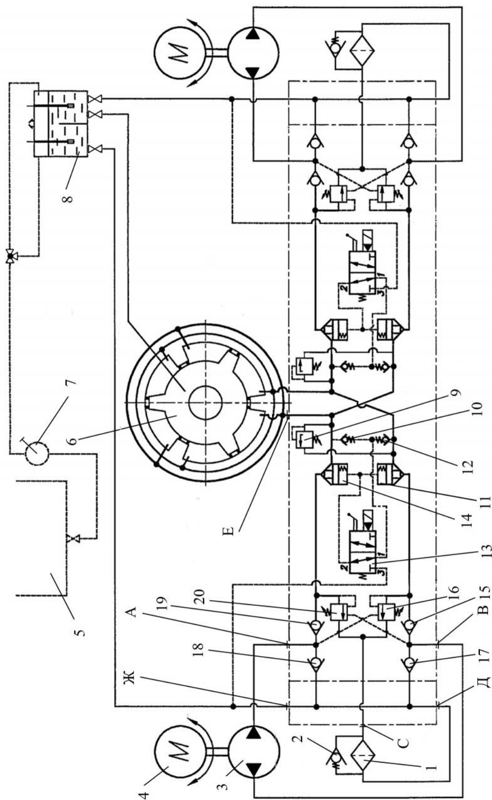
Рис. 8. Принципиальная гидравлическая схема СРМ: 1 – фильтр; 2, 10, 12, 15, 17, 18, 19 – клапан невозвратный; 3 – насос; 4 – электродвигатель; 5 – цистерна запаса РЖ; 6 – рулевая машина; 7 – ручной насос; 8 – расходный бак; 9, 16, 20 – предохранительный клапан; 11, 14 – гидроуправляемый встраиваемый клапан; 13 – гидрораспределитель
