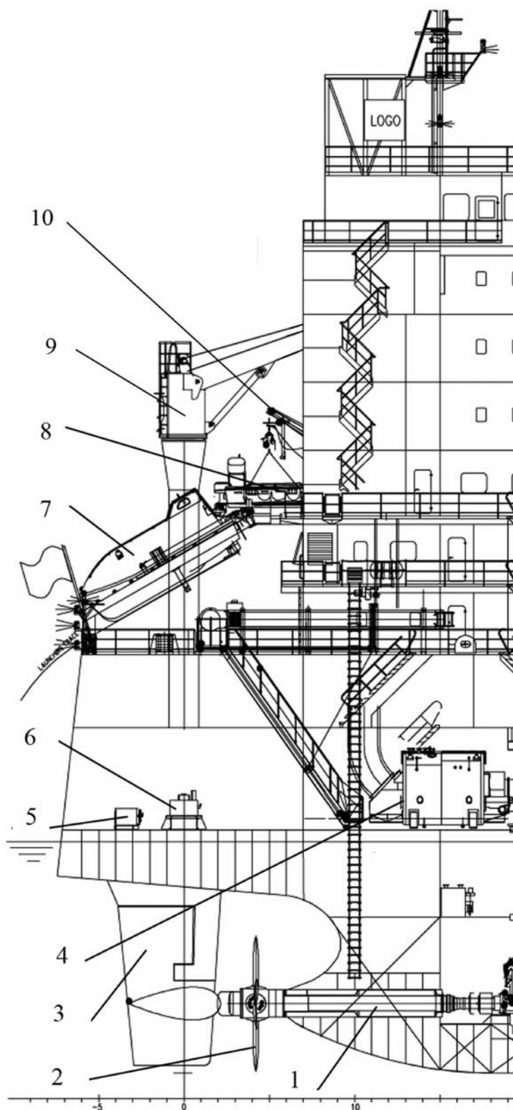
Рис. 1. Общий вид кормовой оконечности контейнеровоза водоизмещением 33700 т (1200 TEU): 1 – валопровод; 2 – винт регулируемого шага; 3 – руль; 4 – комбинированный термомасляный котел; 5 – насосная станция рулевой машины; 6 – рулевая машина; 7 – спасательный катер (22 + 2); 8 – катер (6); 9 – провизионный кран; 10 – кран-балка
