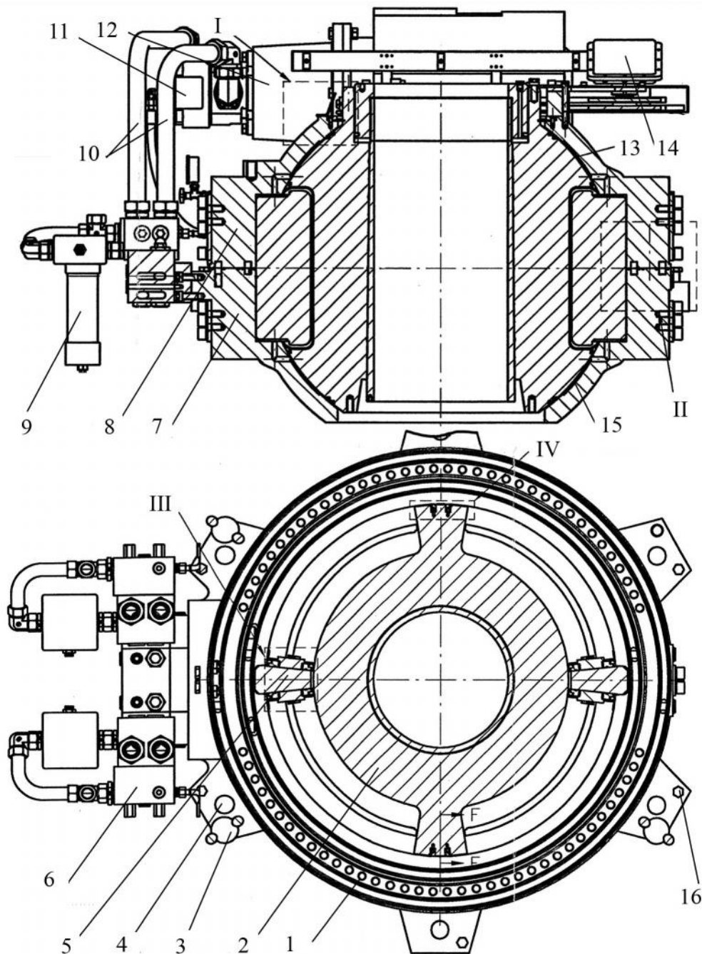
Рис. 5. Внутренне устройство СРМ SV430-2 FCP: 1, 16 – болт; 2 – ротор; 3 – рым-болт; 4 – отверстие; 5 – лопасть статора; 6 – блок гидроаппаратуры; 7, 8 – нижняя и верхняя части статора СРМ; 9 – фильтр; 10 – трубопровод; 11 – насос; 12 – электродвигатель; 13, 15 – верхний и нижний подшипники ротора; 14 – блок контроля угла поворота ротора
