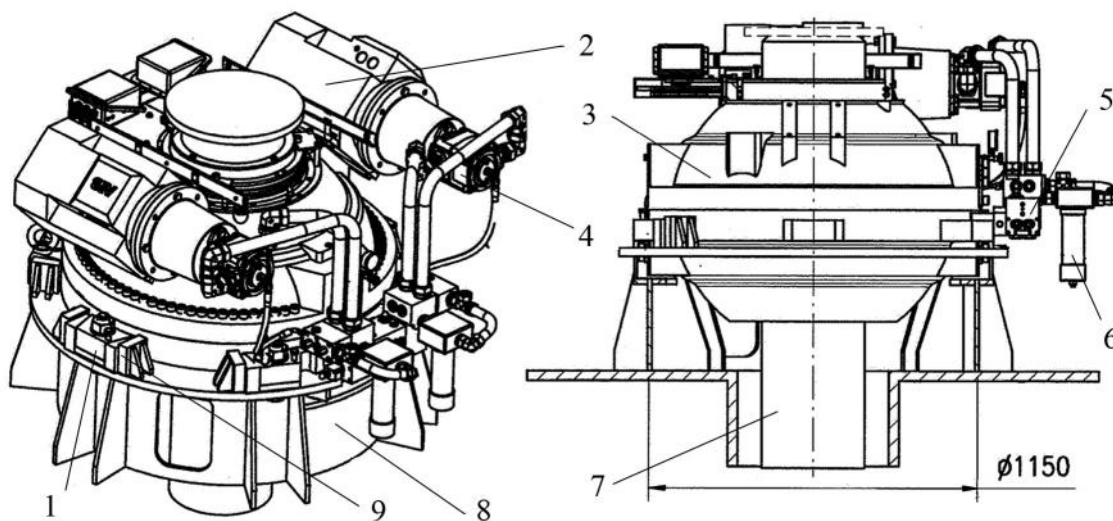
Рис. 4. Общий вид судовой рулевой машины SV430-2 FCP: 1 – упорное ухо рулевой машины; 2 – электродвигатель; 3 – корпус машины; 4 – насос высокого давления; 5 – блок гидроаппаратуры; 6 – фильтр; 7 – баллер; 8 – фундамент; 9 – упорные элементы фундамента
