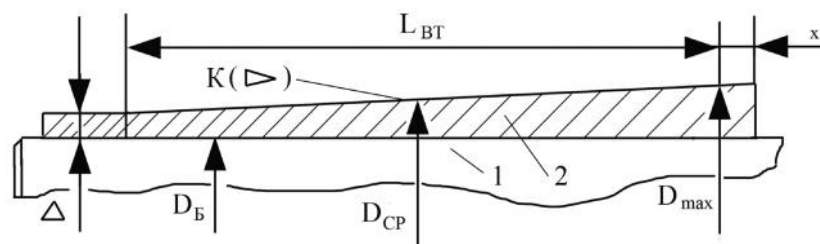
Рис. 16. Схема конической втулки: 1 – баллер; 2 – втулка
