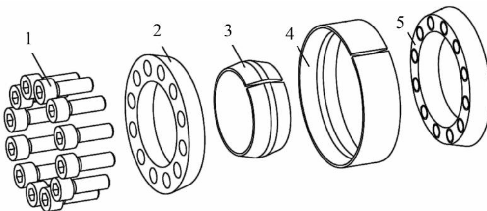
Рис. 12. Последовательность сборки клиновой муфты: 1 – винт; 2, 5 – конические втулки; 3, 4 – разрезные конические кольца
