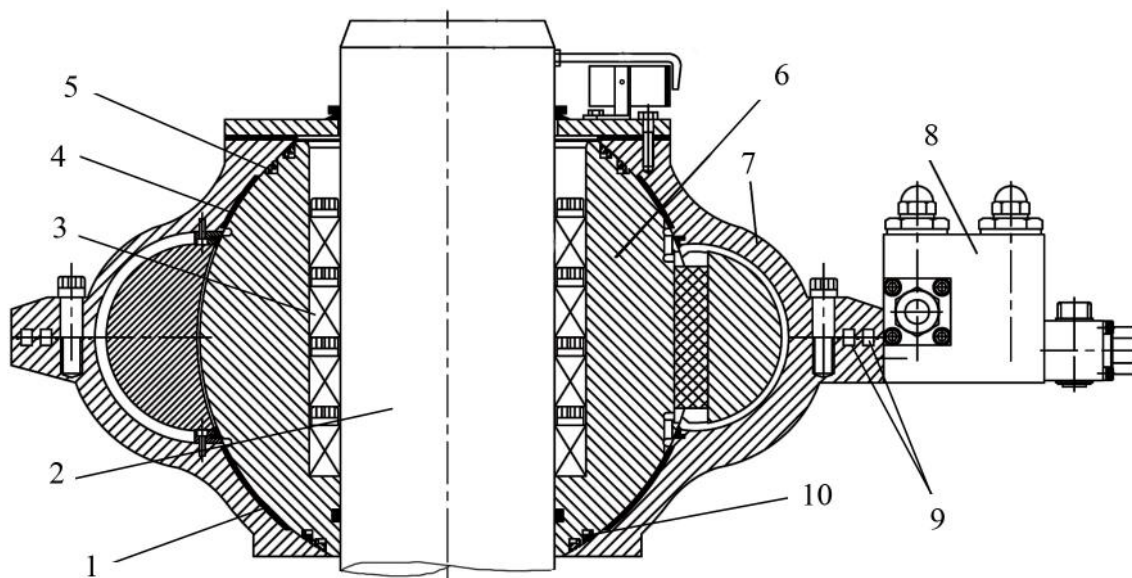
Рис. 10. Соединение ротора посредством клиновых колец: 1, 4 – подшипники скольжения; 2 – баллер; 3 – клиновые кольца; 5, 9 – уплотнения; 6 – ротор; 7 – корпус машины; 8 – гидроблок; 9 – каналы подачи РЖ
