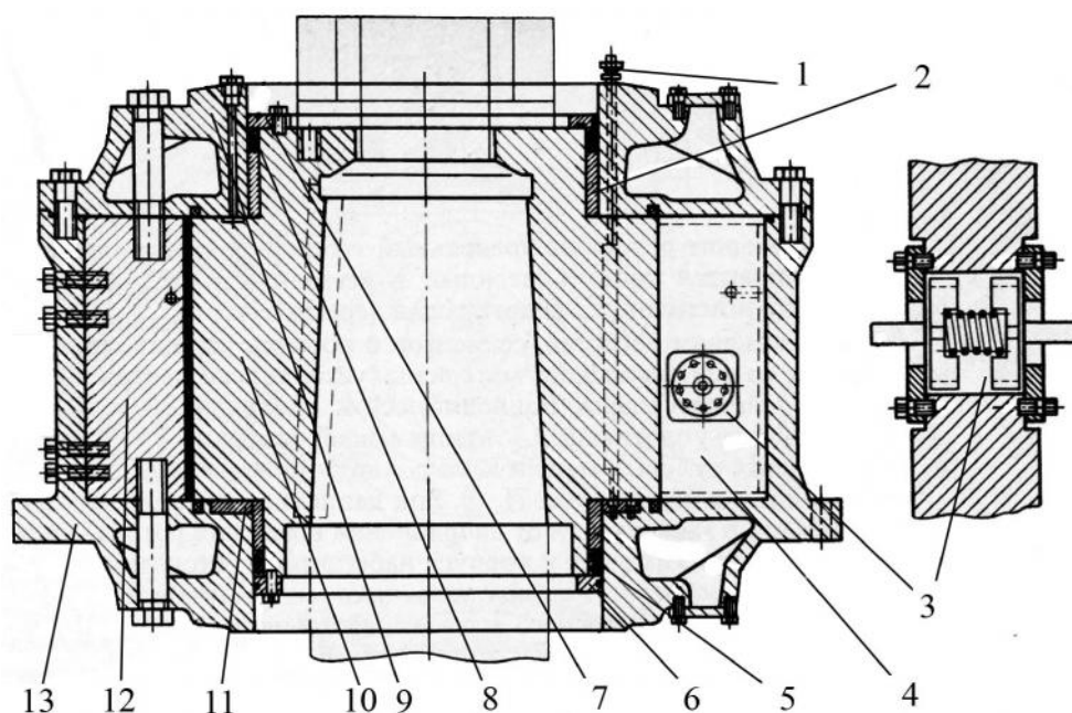
Рис. 3. Устройство лопастной рулевой машин: 1 – штуцер; 2 – радиальный подшипник; 3 – предохранительный клапан; 4 – лопасть; 5, 8 – сальник; 6, 7 – нажимные фланцы; 9 – крышка; 10 – ротор; 11 – опорно-упорный подшипник; 12 – неподвижная лопасть; 13 – корпус
