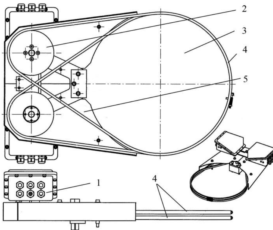
Рис. 7. Устройство электромеханической обратной связи: 1 – корпус командоаппарата; 2 – ведомая звездочка; 3 – корпус рулевой машины; 4 – цепи; 5 – защитный чехол
