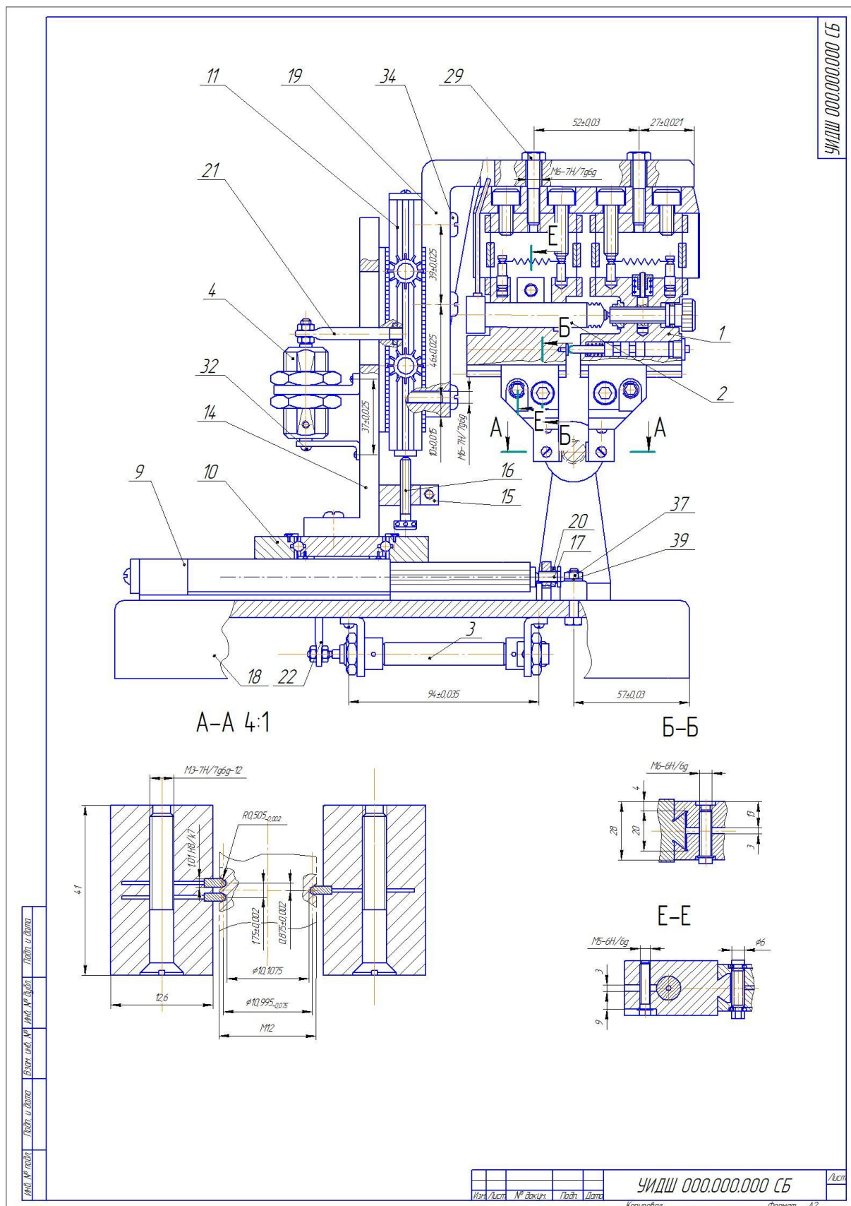
Рисунок А.6 – Измерительная станция (сборочный чертеж) (лист 2)
