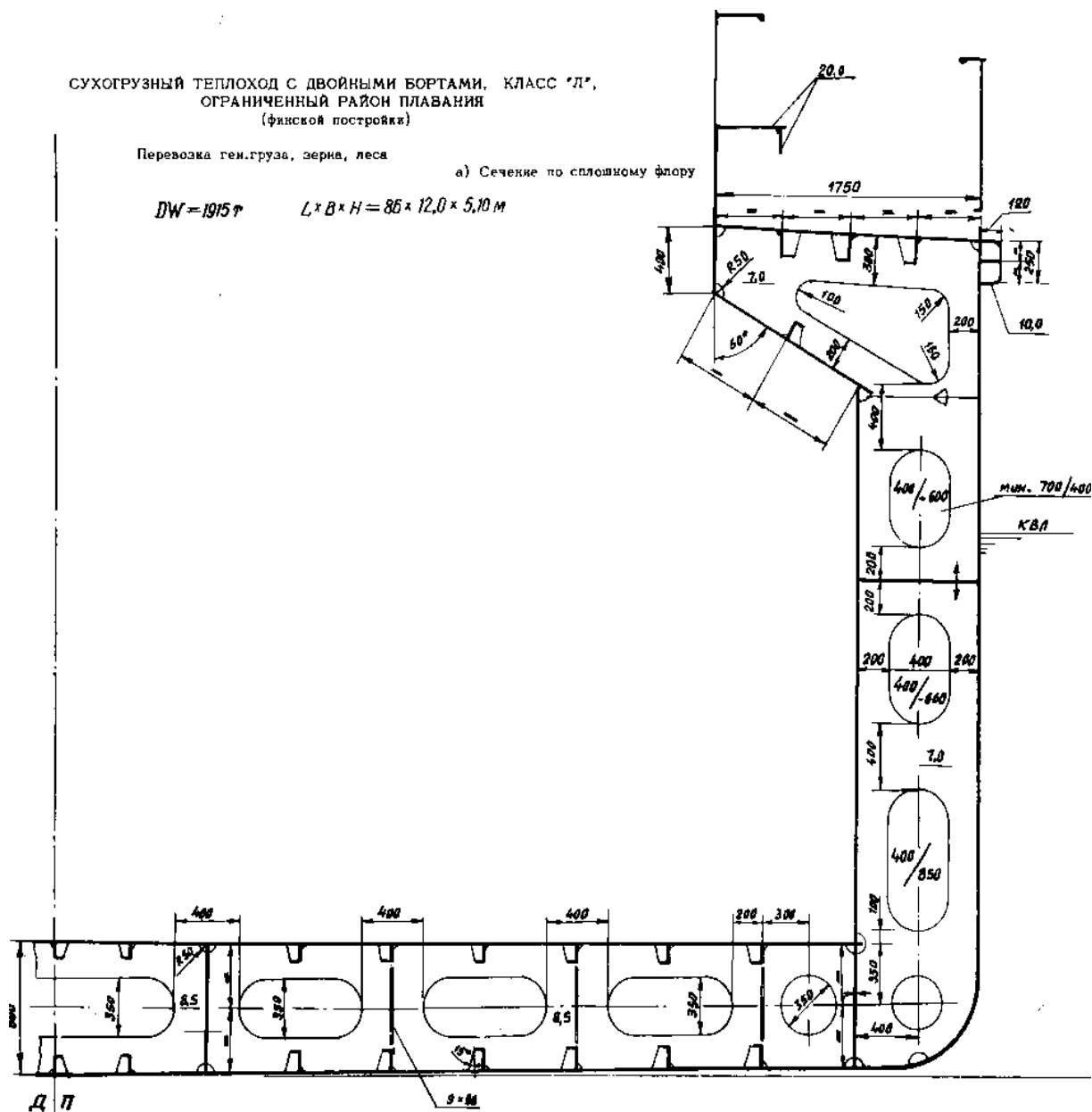
Рис. Б.2. Эскиз мидель-шпангоута сухогрузного судна
