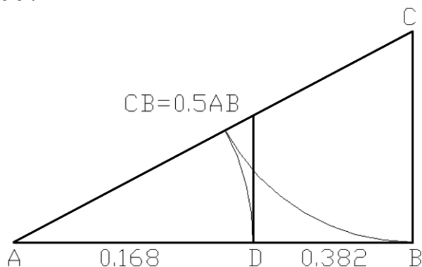
Рис. 4. Построение «Золотого сечения»
