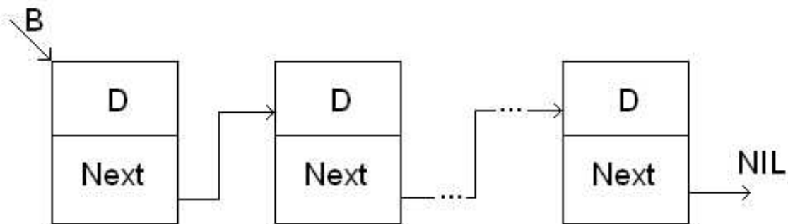
Рисунок 7.2 — Связный однонаправленный список
