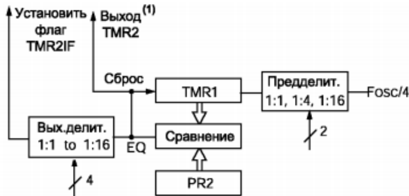
Рис. 5.6 — Структурная схема модуля TMR2
