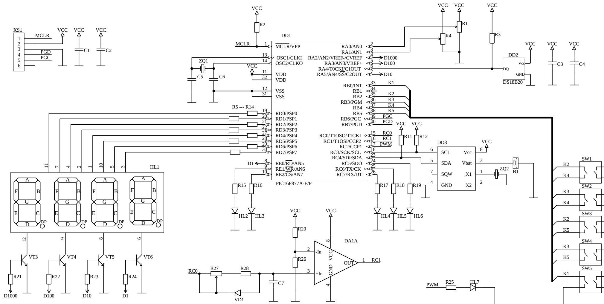
Рис 1.1 — Электрическая принципиальная схема макета на базе микроконтроллера PIC16F877
