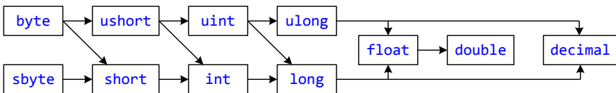
Рис. 2.1 – Схема неявного преобразования числовых типов.
