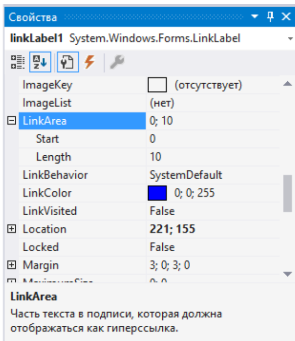
Рис. 3.5 – Свойство элемента LinkLabel : LinkArea
