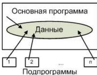
Рис. 2 – Архитектура программы с глобальной областью данных
