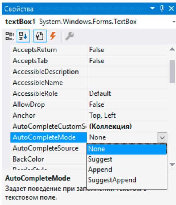
Рис. 3.8 – Опции настройки AutoCompleteMode
