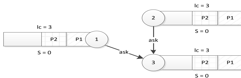
Рис. 1.11 – Размещение Р-сообщения в очереди. Подтверждение принятия Р-сообщения
