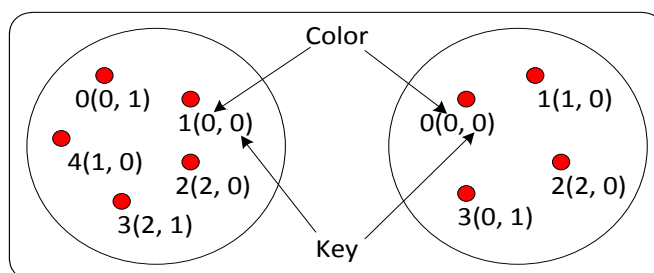
Рис. 1.11 – Входной коммуникатор ( comm )
