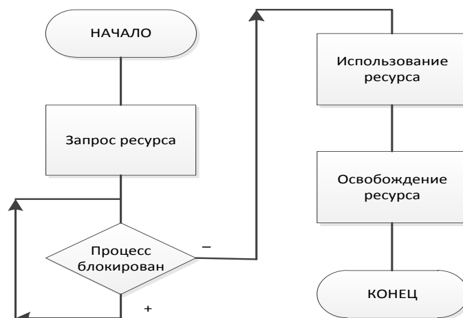
Рис. 1.3 – Алгоритм функционирования клиента
