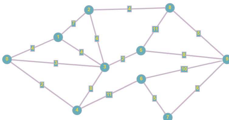
Рис. 2.1 – Исходный граф для реализации алгоритма Дейкстры
