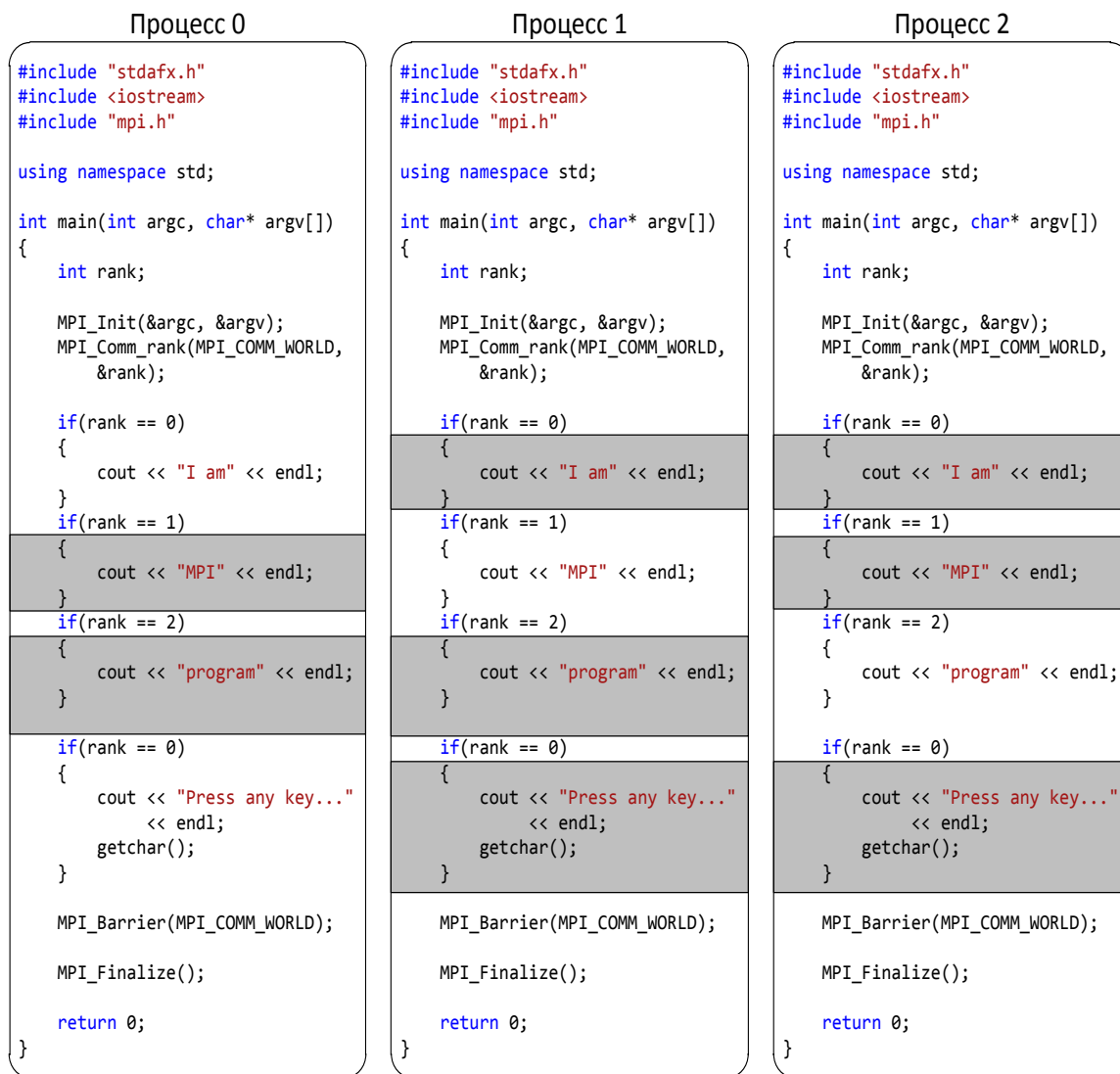
Рис. 1.5 – Пример ветвления при организации выполнения процессов
