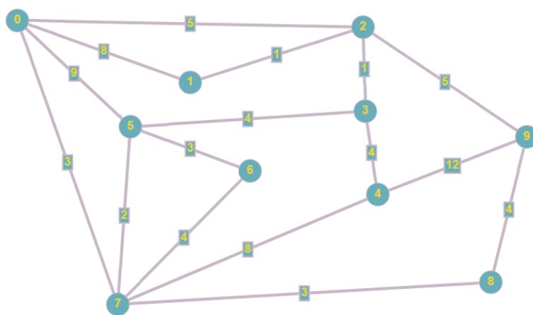
Рис. 2.3 – Исходный граф для реализации алгоритма Крускала
