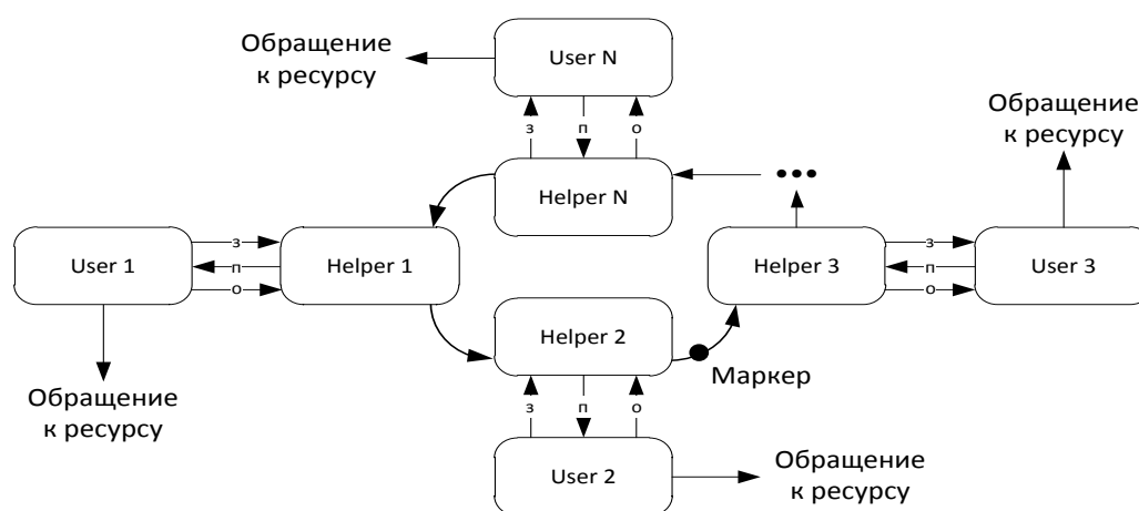
Рис. 1.14 – Реализации алгоритма передачи маркера
