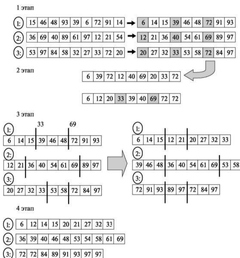
Рис. 1.14 — Пример работы алгоритма сортировки с использованием регулярного набора образцов
