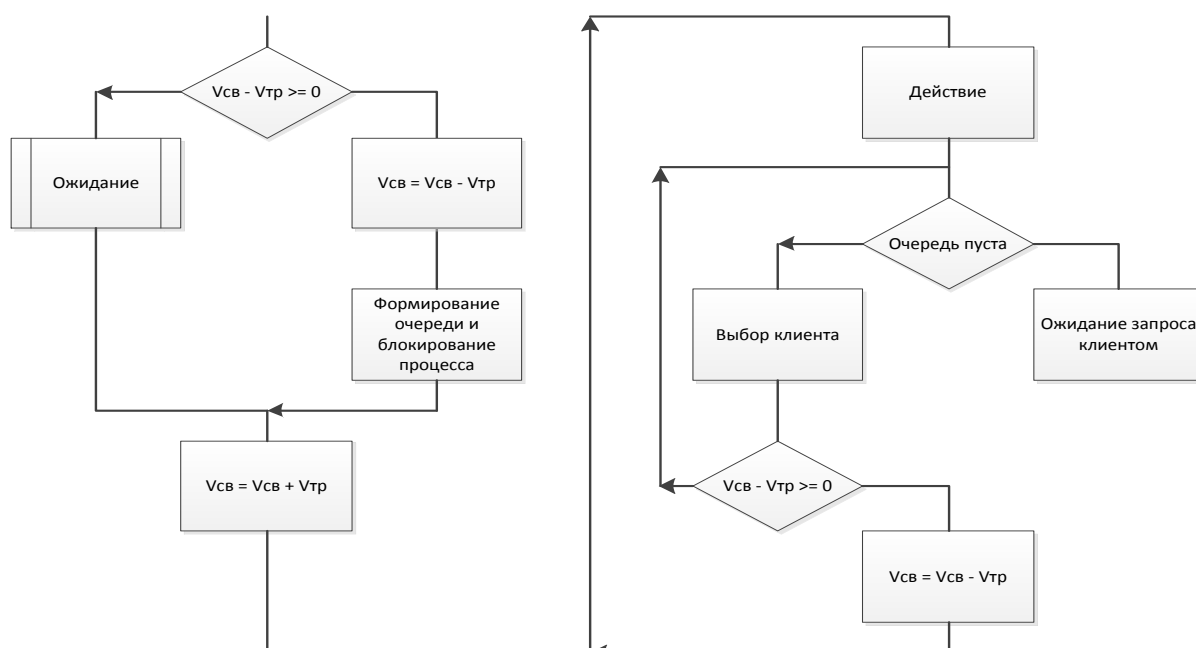
Рис. 1.8 –Фрагмент алгоритма контроля информационных структур сервера при запросе и освобождении ресурса
