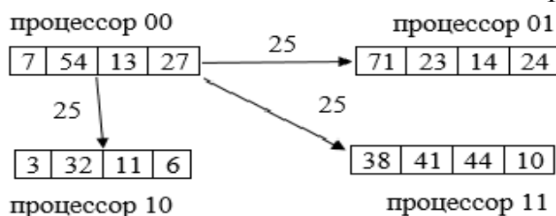
Рис. 1.2 — Распределение данных и опорного элемента по ПЭ
