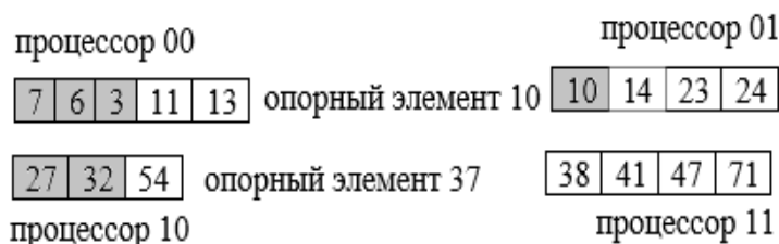
Рис. 1.6 — Результат разделения на подмассивы относительно опорного элемента
