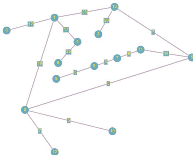
Рис. 2.3 – Исходный разрешенный граф для реализации алгоритма Белмана-Форда
