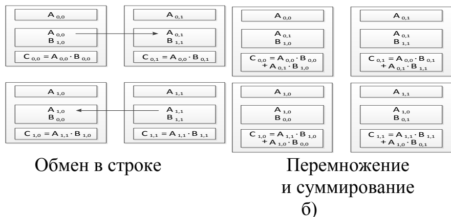
Рис. В.4 – Состояние блоков в каждой подзадаче в ходе выполнения итераций алгоритма Фокса: а) первая итерация алгоритма; б) вторая итерация алгоритма
