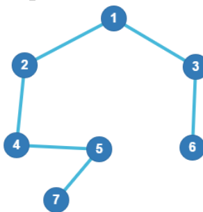
Рис. 1.2 — Результирующий граф
