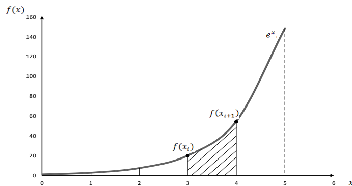
Рис. 2.2 – Частичная сумма интеграла
