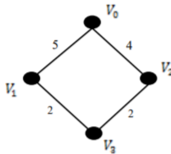
Рис. 1.1 — Исходный граф
