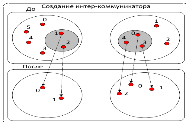
Рис. 1.10 – Создание интер-коммуникатора
