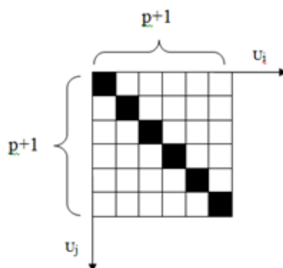
Рис. 1.4 — Сетка процессов и формирование подматриц весов
