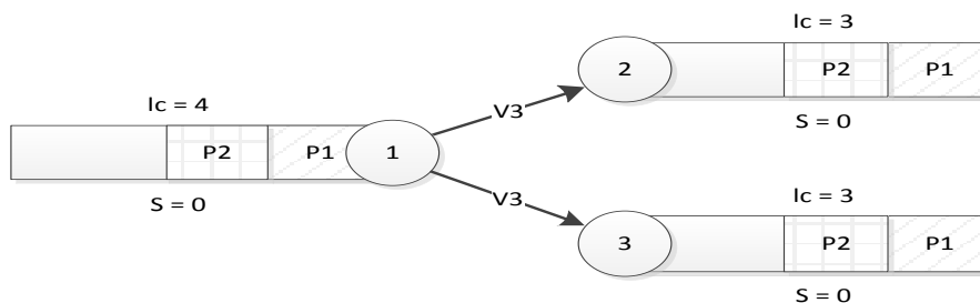
Рис. 1.12 – Обработка третьим процессом значения переменной S. Посылка первым процессом сообщения V об освобождении ресурса
