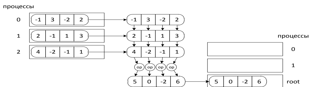
Рис. 1.9 – Пример выполнения операции редукции
