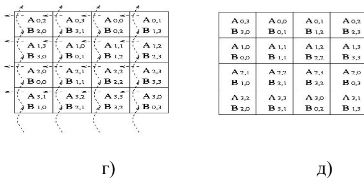
Рис. В.5 – Состояние блоков в каждой подзадаче в ходе выполнения итераций алгоритма Фокса при q=4 :
