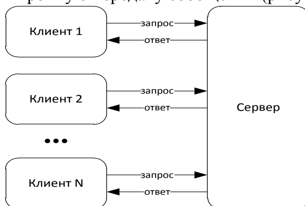
Рис. 1.1 – Схема взаимодействия типа «клиент-сервер»
