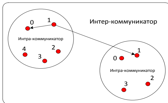
Рис. 1.1 – Интра- и интер-коммуникаторы
