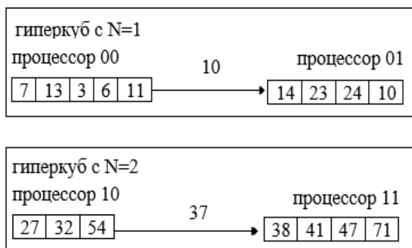
Рис. 1.5 — Широковещательная рассылка опорного элемента
