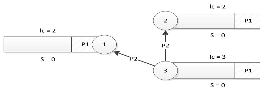
Рис. 1.10 – Запрос третьим процессом ресурса. Отправка сообщения с идентификатором Р-операции
