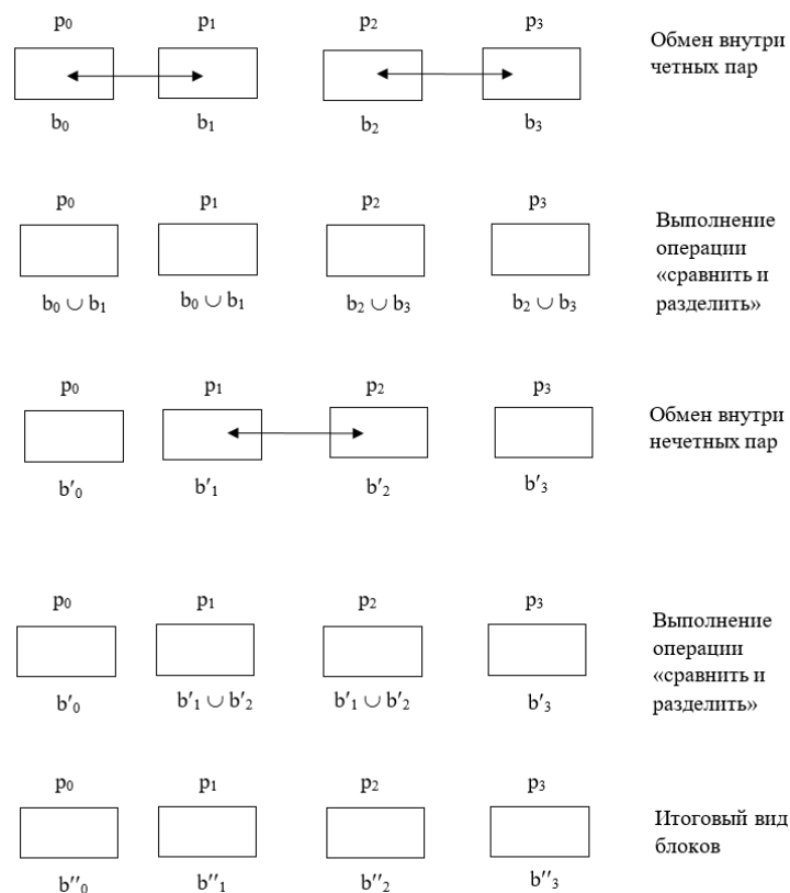
Рис. 1.2 – Схема реализации четно-нечетной перестановки при P < n
