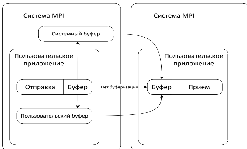
Рис. 1.2 – Использование буферов при реализации обмена
