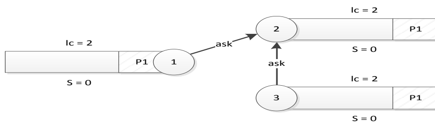
Рис. 1.9 – Размещение полученного сообщения в очереди, подтверждение приемниками получения сообщения сигналом ask
