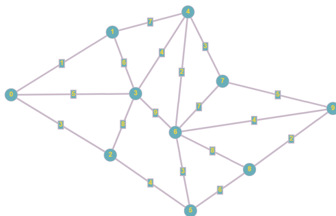
Рис. 2.2 – Исходный граф для реализации алгоритма Белмана-Форда
