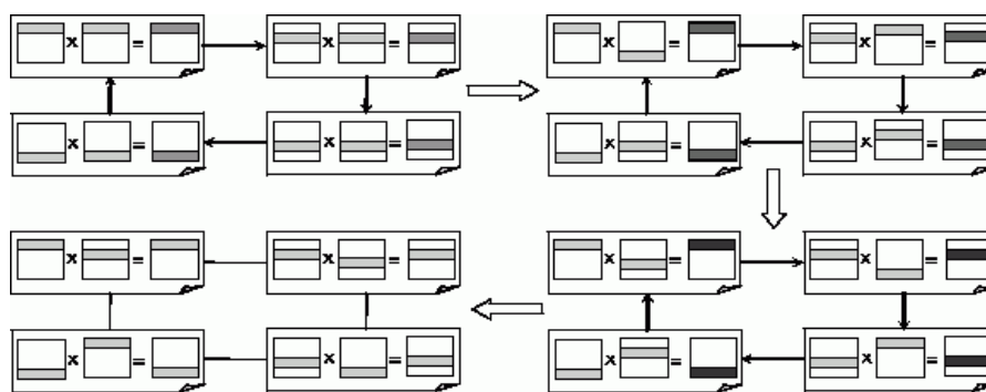
Рис. В.3 – Схема передачи данных для второго параллельного алгоритма матричного умножения (ленточная схема разделения данных)
