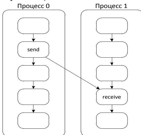
Рис. 1.1 – Взаимодействие процессоров типа «точка-точка»
