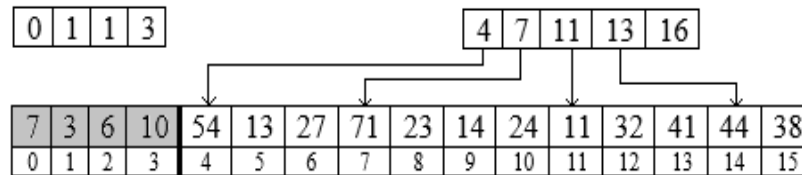
Рис. 1.10 — Результирующая последовательность (первый этап)
