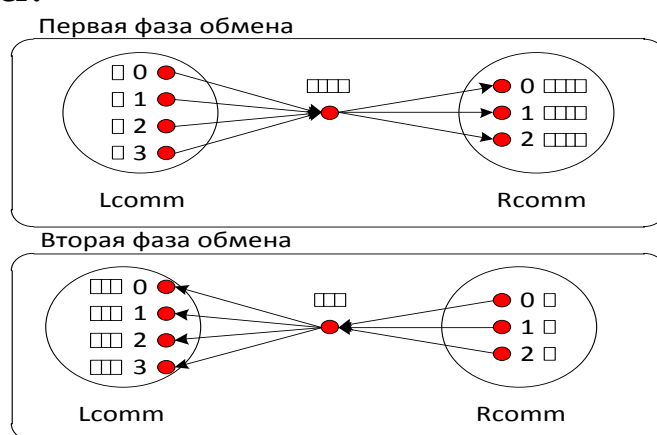
Рис. 1.2 – Интер-коммуникатор allgather
