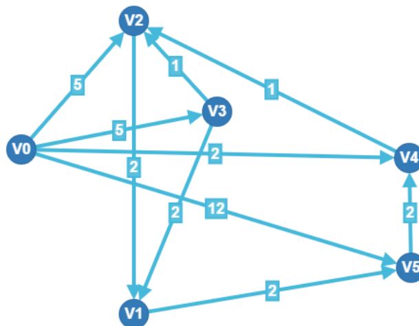
Рис. 1.3 — Исходный граф
