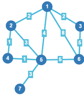
Рис. 1.1 — Исходный граф
