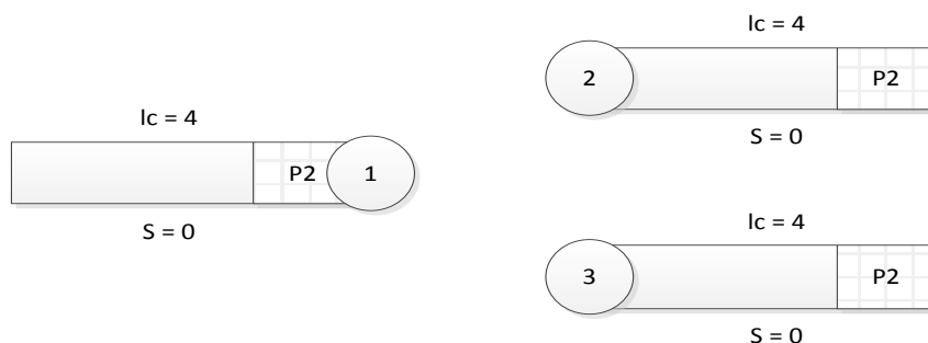
Рис. 1.13 – Обработка очереди
