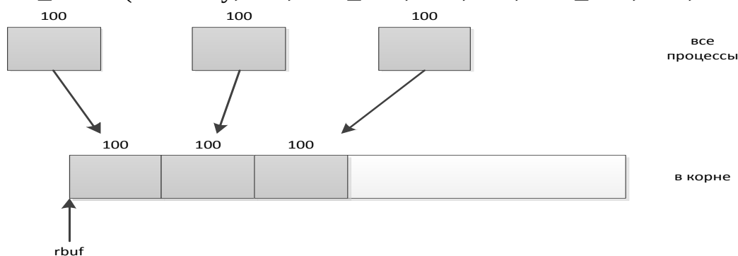
Рис. 1.5 – Схема реализации сбора значений
