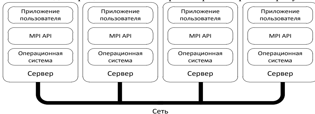
Рис. 1.2 – Вычислительная система с четырьмя рабочими станциями
