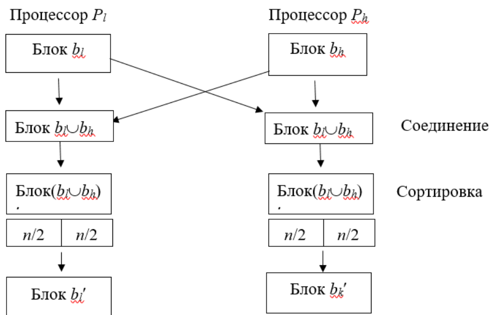
Рис. 1.1. – Схема реализации процедуры «сравнить и разделить»
