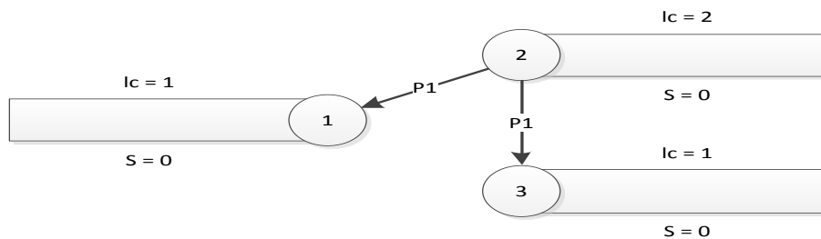
Рис. 1.8 – Запрос вторым процессом ресурса. Отправка сообщений с идентификатором Р-операции
