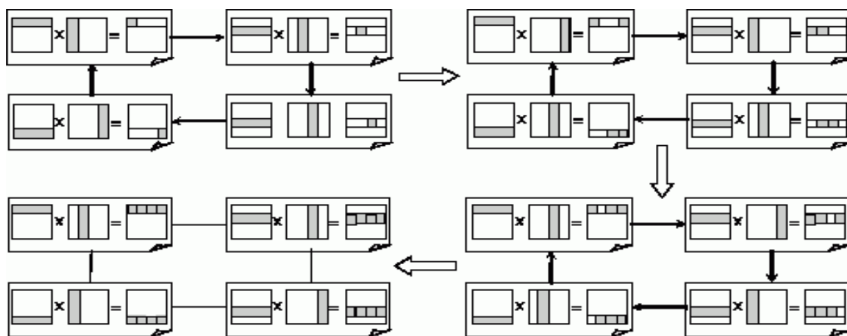
Рис. В.2 – Схема передачи данных для первого параллельного алгоритма матричного умножения (ленточная схема разделения данных)
