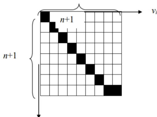
Рис. 1.5 — Разбиение матрицы смежности W(v_i, v_j) на подматрицы для разрешенного графа
