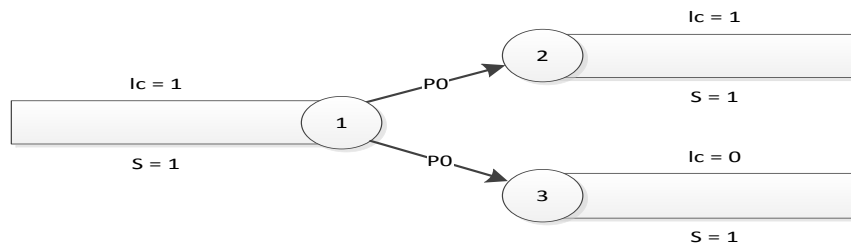
Рис. 1.5 – Запрос захвата ресурса первым процессом
