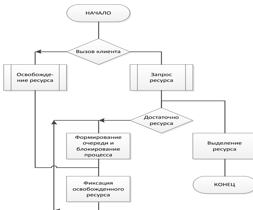
Рис. 1.2 – Алгоритм функционирования сервера
