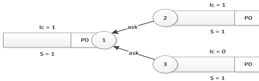
Рис. 1.6 – Размещение сообщения P0 в очереди и отсылка подтверждающих сообщений ask (логические часы при принятии P-сообщения увеличиваются на 1)
