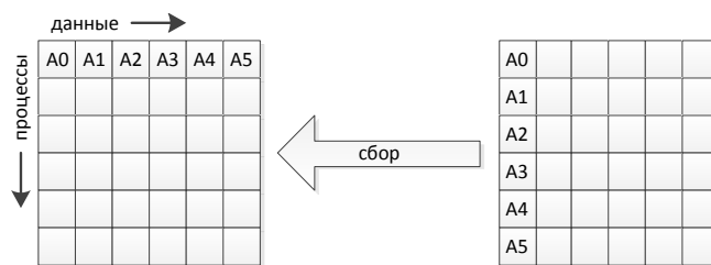
Рис. 1.4 – Иллюстрация функции сбора
