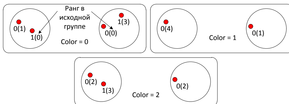
Рис. 1.12 – Отделенные выходные коммуникаторы ( newcomm )
