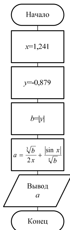
Рисунок 2.5 – Схема алгоритма вычислений
