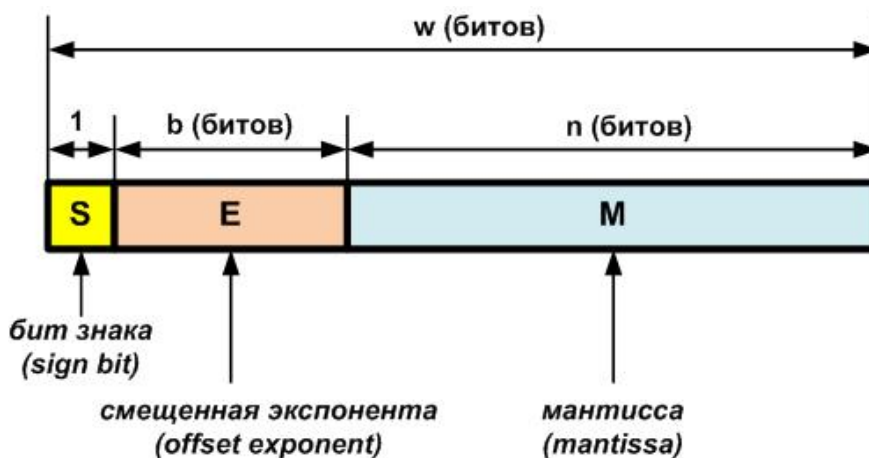
Рисунок 5.1 – Формат IEEE-754
