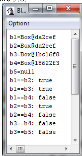
Рисунок 3.6 – Результаты работы программы при отсутствии в классе Box метода toString ()
