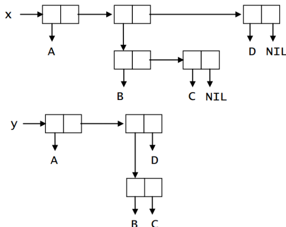
Внутреннее представление списочных структур
