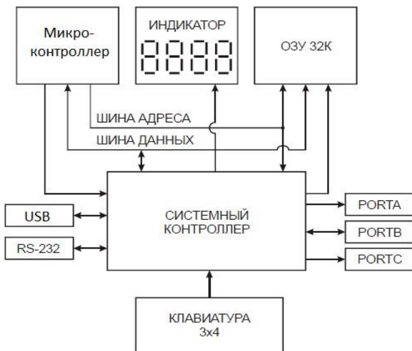
Рис. 1.4 — Структурная схема основного модуля отладочного стенда
