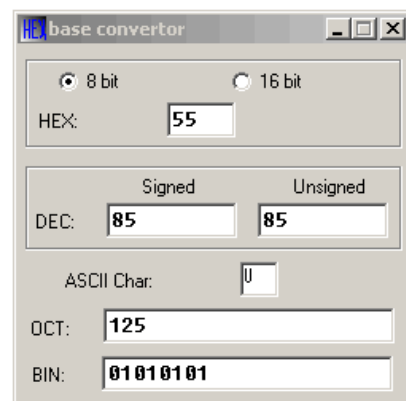
Рисунок 3.5 – Окно конвертера
