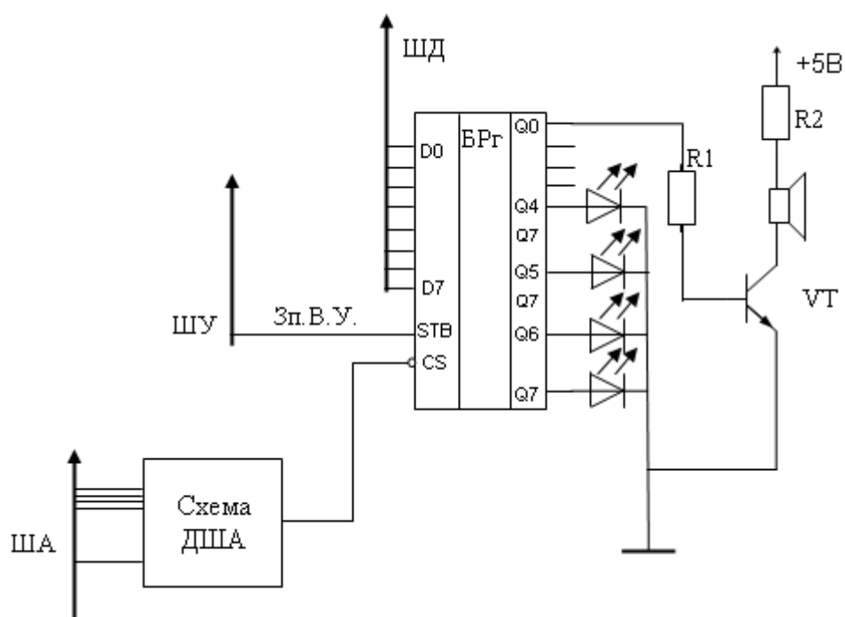
Рисунок 2.2 — Схема выходного устройства, построенного на базе буферного регистра (БРг) со светодиодами и динамиком
