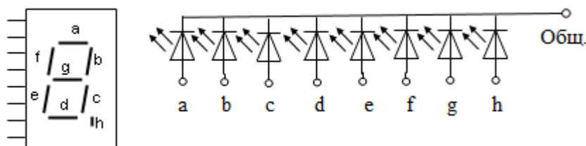
Рисунок 2.3 — Внешний вид и схема семисегментной светодиодной матрицы
