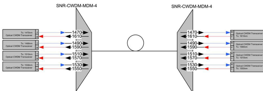
Рис. 2.19 — Схема применения оптических мультиплексоров для CWDM -уплотнения
