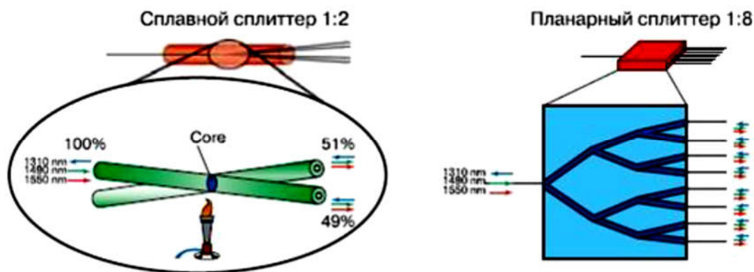
Рис. 2.9 — Основные технологии изготовления оптических сплиттеров
