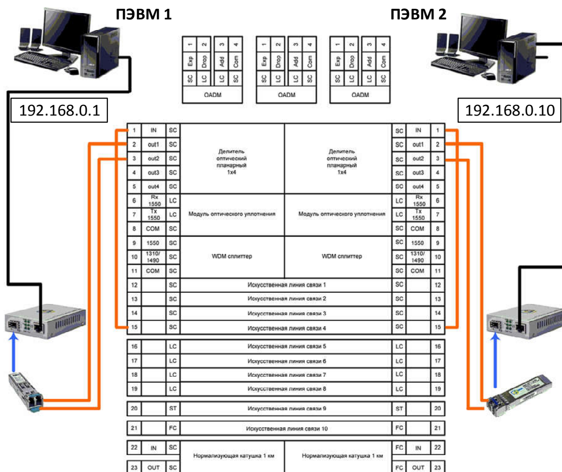
Рис. 2.12 — Сеть с WDM -уплотнением на базе широкополосных сплиттеров
