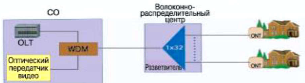
Рис. 2.10 — Упрощённая структурная схема сети PON с планарным Y-образным оптическим разветвителем
