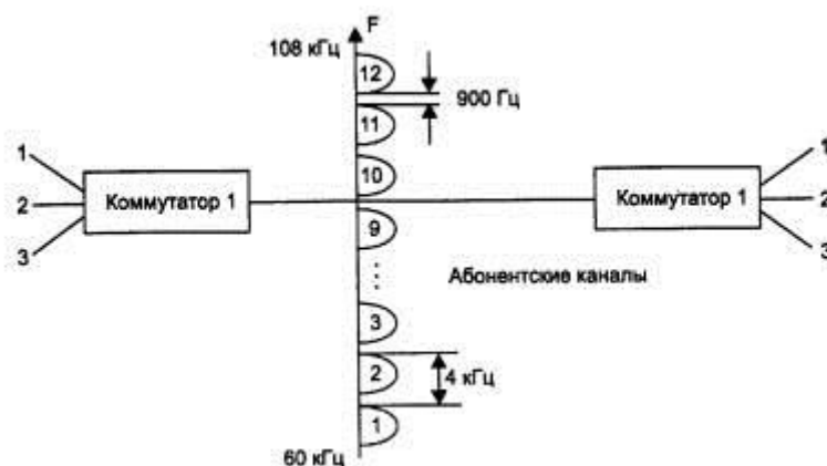
Рис. 3.15 — Коммутация на основе частотного уплотнения
