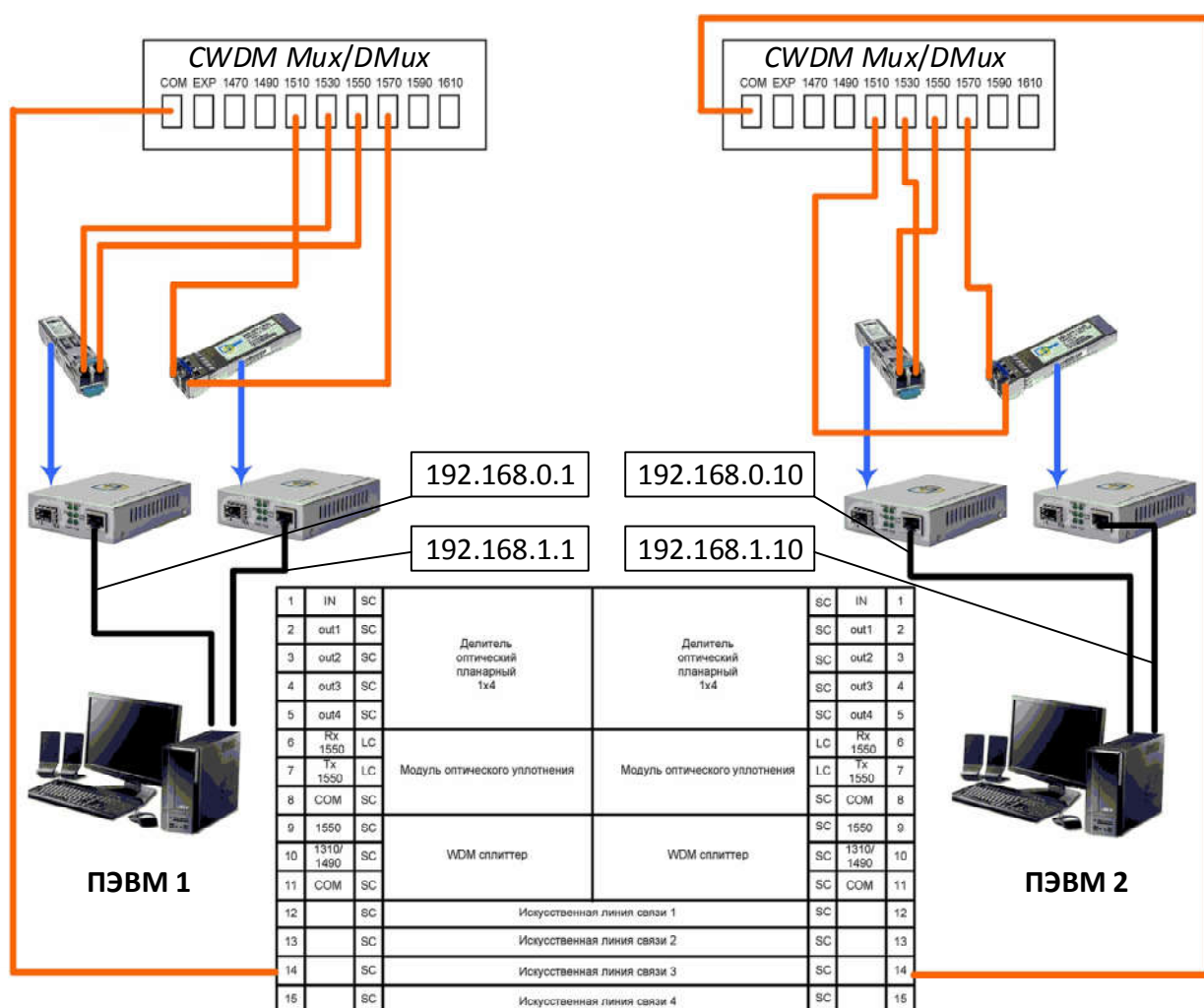
Рис. 2.23 — Схема сети с CWDM -уплотнением
