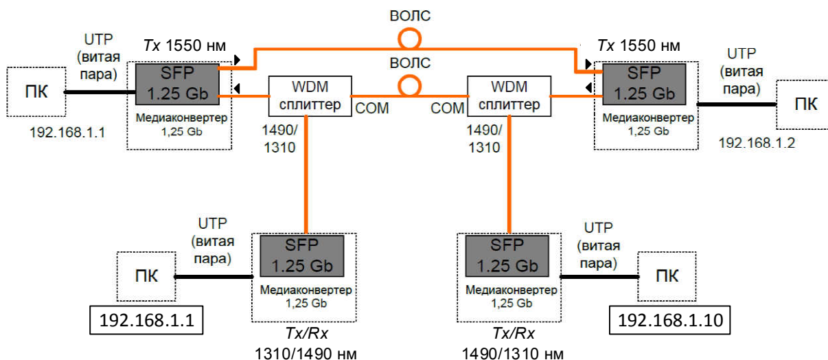
Рис. 2.7 — Схема сети с WDM -уплотнением на базе оптических WDM -сплиттеров
