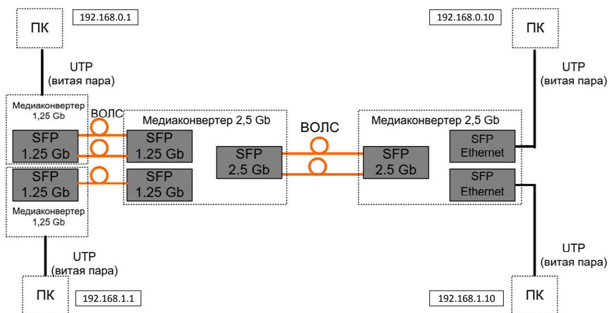
Рис. 3.17 — Топология сети с TDM уплотнением
