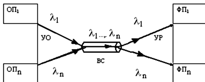
Рис. 2.1 — Принципиальная схема волнового (спектрального) уплотнения)
