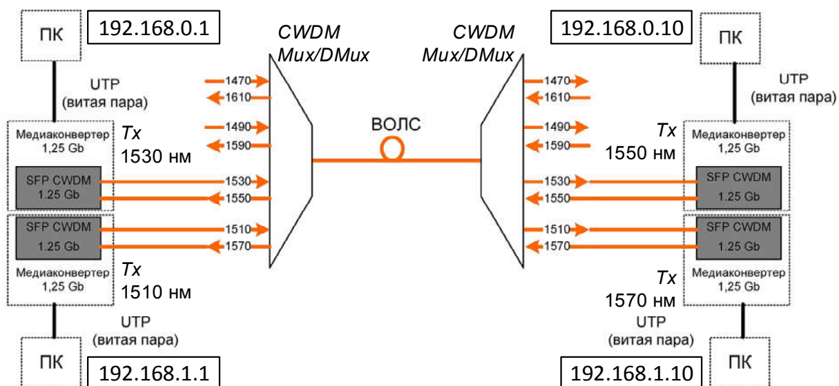
Рис. 2.22 — Структурная схема сети с CWDM -уплотнением
