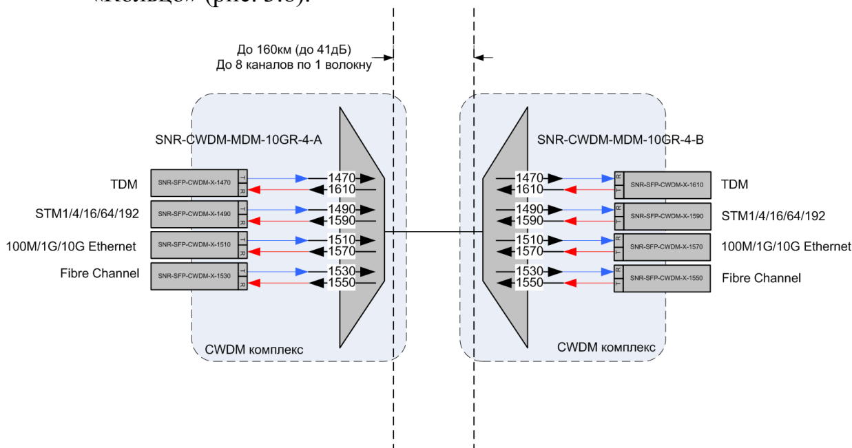
Рис. 3.6 — Топология «точка-точка»
