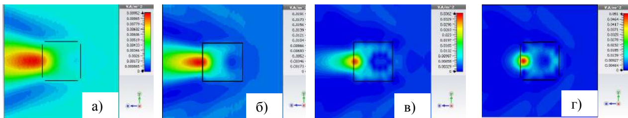
Рис. 1. Распределение электромагнитного поля в ближней зоне диэлектрического куба 7x7 мм на частоте 42 ГГц: а) n=1,2 ; б) n=1,41 ; в) n=1,73 ; г) n=2,00 .
