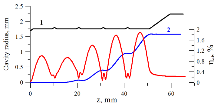
Рис. 2. Гиротрон с секционированным резонатором на четвертой циклотронной гармонике. Оптимизированный профиль резонатора (кривая 1) и структура поля рабочей моды TE_{4,5} , а также рассчитанная зависимость электронного КПД от продольной координаты (кривая 2).
