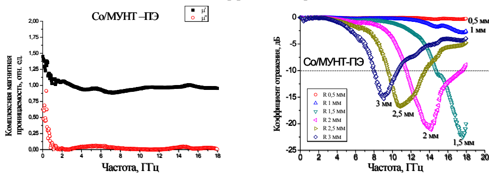
Рис. 1. Частотные зависимости комплексной магнитной проницаемости и коэффициента отражения при расположении материала на проводящей поверхности
