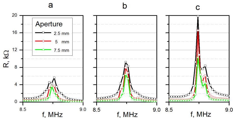
Рис. 2. Частотная зависимость реальной части импеданса A1 волны при различных значениях апертуры и количества пар ВШП: (a) 7 пар, (b) 5 пар, (c) 3 пары.
