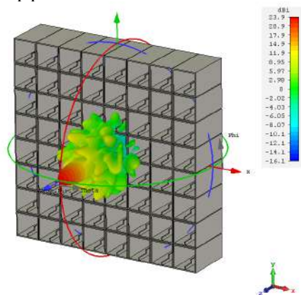
Рис.1. Антенная решетка из волноводных излучателей с круговой поляризацией
