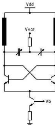
Рисунок 1 — Упрощенная принципиальная схема ГУН
