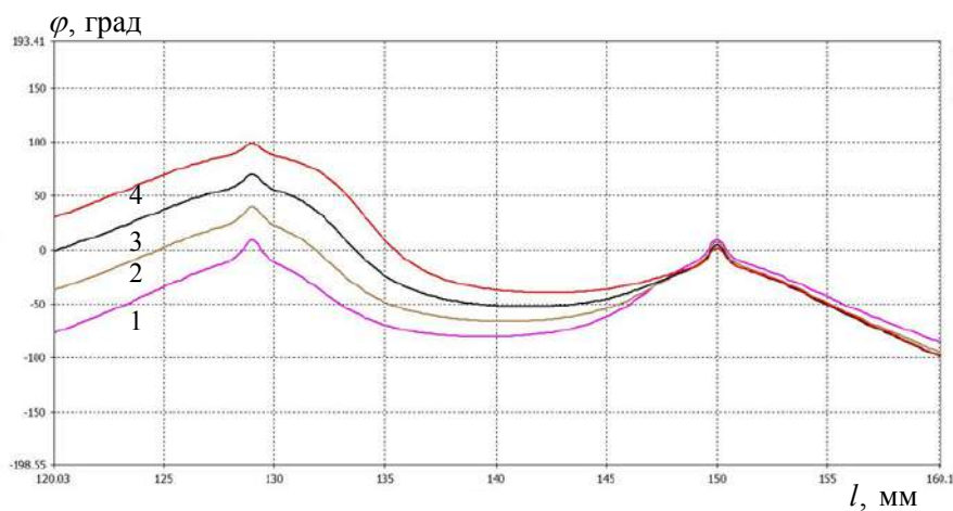
б) поведение фазы поля в промежутке между диполями
