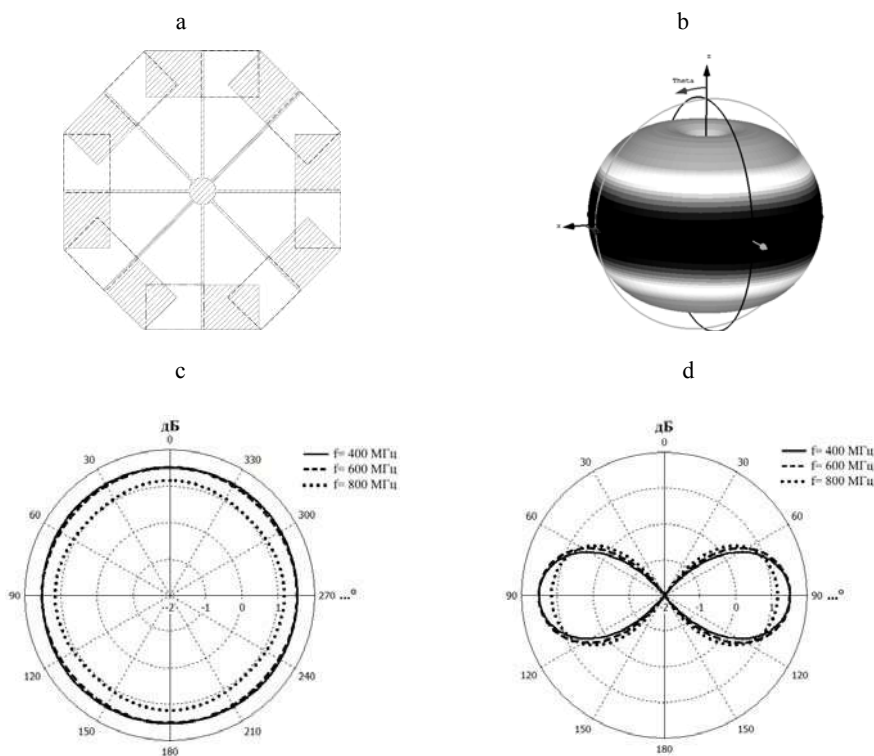
Рис. 2. Вид излучателя (а), 3D ДН (б), ДН в азимутальной плоскости (с) и ДН в угломерной плоскости (д)
