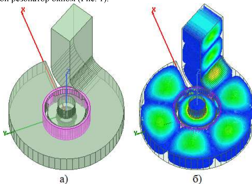
Рис. 1. Конструкция вывода энергии СМК с интегрированным с выходным резонатором окном (а) и распределение электрического поля на рабочей частоте f=2.856 ГГц (б).
