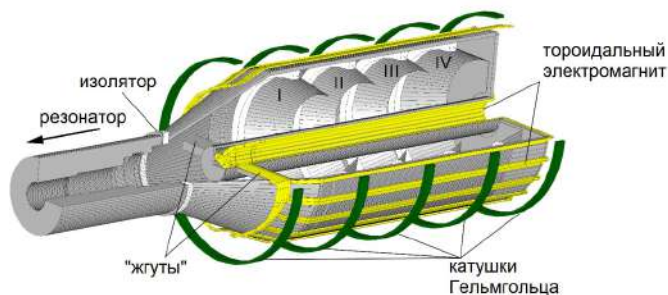
Рис. 1. Схематическое изображение модели коллектора. I-IV – секции коллектора.
