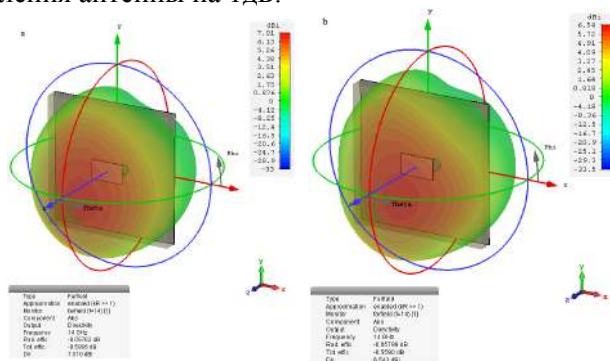
Рис.4. Пространственные диаграммы направленности печатных излучателей без распределенного возбуждения (а) и с распределенным возбуждением (б).
