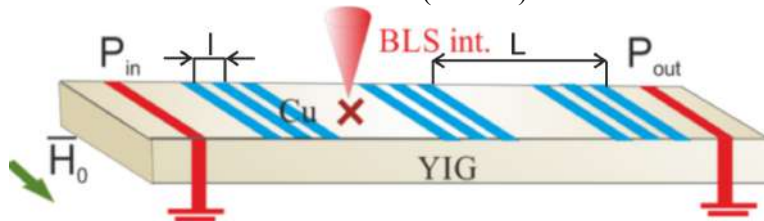
Рис. 1. Схема суперрешетки на основе 1-D магнитного кристалла.
