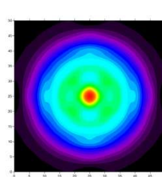
Рис.3. Распределение поля на внешнем квазиоптическом зеркале \eta=98,2\% .
