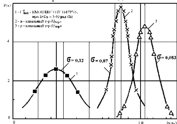
Рисунок 2. Распределения усредненных по пластине U_{\text{вых}}^0 чипов КМОП БИС ОЗУ 1617РУ6 от дозы (1), Упор n- и p- канальных МОП транзисторов (2, 3), полученные на ускорителе электронов с E_e = 130 кэВ
