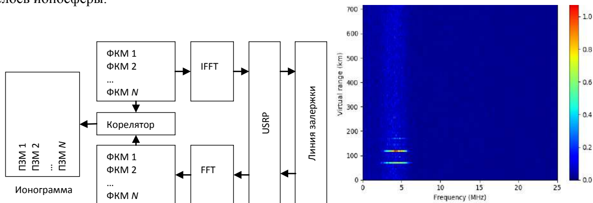
Рис. 1 Структурная схема тестирования OFDM ионозонда (слева) и симулированная с помощью линии задержки ионограмма, полученная с помощью OFDM ионозонда (справа)
