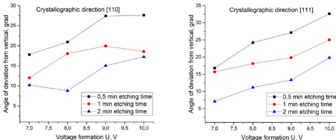
Рис. 2. Зависимость угла отклонения от вертикали от напряжения формирования маскирующего покрытия и различных временах плазмохимической обработки а) кристаллографическое направление [110]; б) кристаллографическое направление [111]
