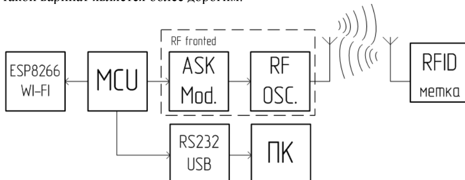
Рис. 1. Структурная схема системы формирования инициирующего возбуждения по протоколу GEN2.
