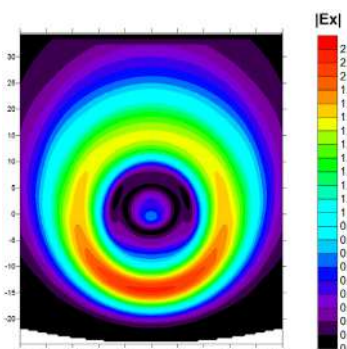
Рис.2. Распределение поля на поворотном зеркале. Вид вдоль оси gyro-ЛБВ.
