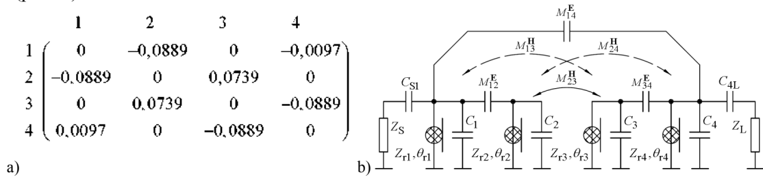
Рис. 2. Матрица связи предложенного КЭФ на МКБ (а) и его эквивалентная схема (б)
