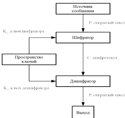
Рисунок 1. Обобщенная схема криптосистемы.
