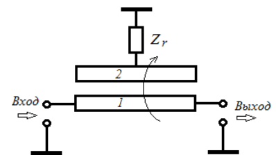
Рис. 1. Эквивалентная схема управляемой секции связанных полосковых линий: 1 – токонесущая полоска; 2 – управляющая полоска; Z_r – сопротивление регулирующего элемента
