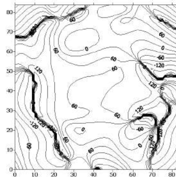
Рис. 3. Восстановленная фаза волнового пучка методом PSO.
